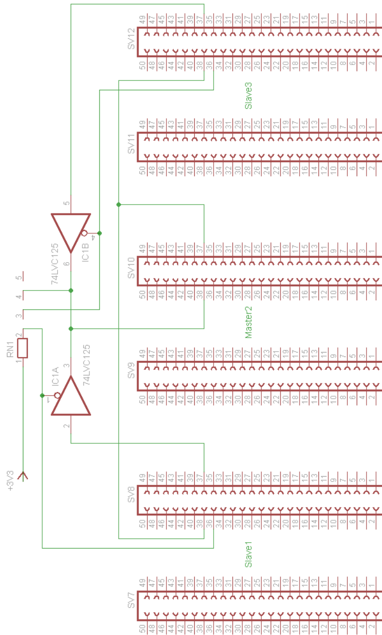
Abbildung 2.2: Kommunikation - Bus
